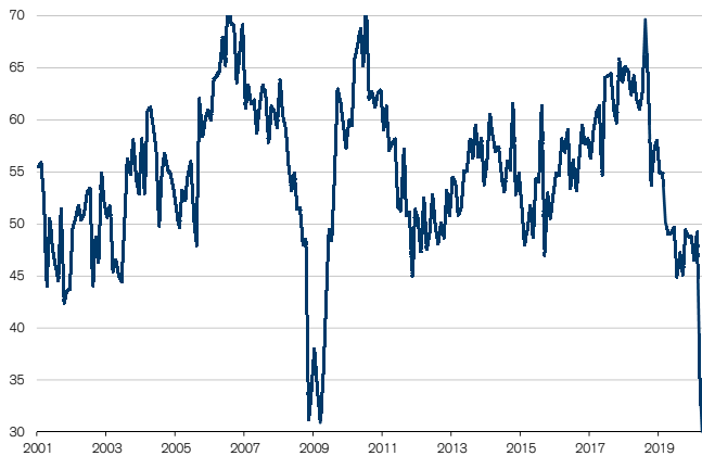
Fig. 2: La production se ressaisit
