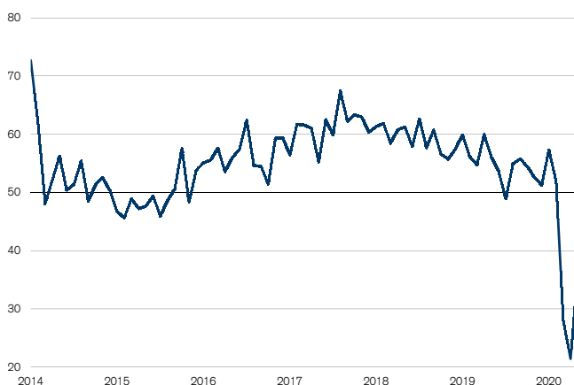
Fig. 3: Les hauts et les bas du PMI services
